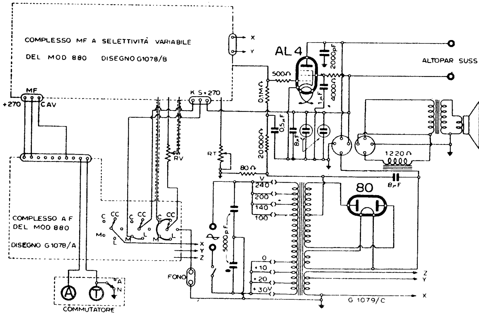
F.I.M.I. - MOD. PHONOIA « 900 » - PARTE BF (AF e MF dell'« 880 »)
